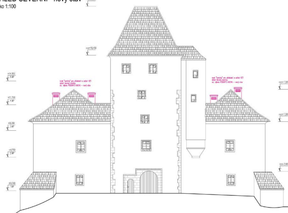
Hlucká Tvrz - Zaměření stávajícího stavu objektu POHLED SEVERNÍ - nový stav měřítko 1:100
