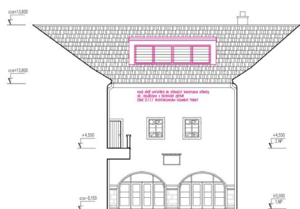
Revitalizace objektu hlucká tvrz POHLED SEVERNÍ - NÁDVOŘÍ - nový stav měřítko 1:100
